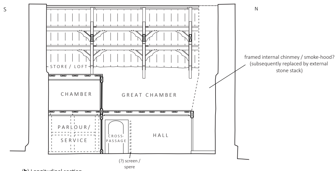
(b) Longitudinal section
